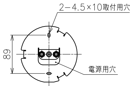
取付板詳細 S:1/5
